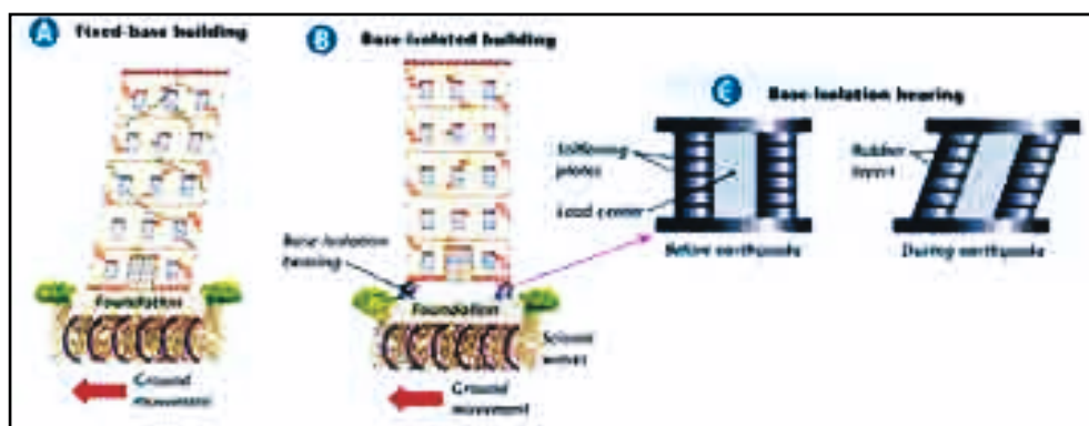
شكل ( ٤ ) أسلوب البناء المقاوم للزلازل
