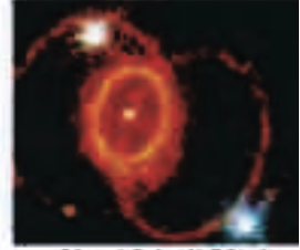
الحلقة الغامضة العميقة بنجم (سوبرنوفا)
