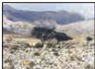
شكل (٢٠) منخفض صحراوي
