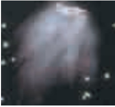
شكل (٩) نيزك
