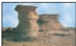
شكل (٢١) موائد صحراوية
