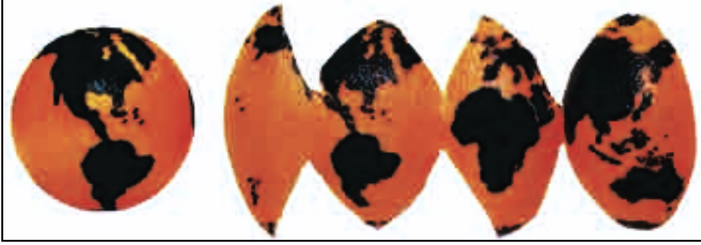
شكل ( ١ ) إسقاط الجسم الكروي
