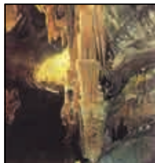
شكل (١٠) كهف الكارست
